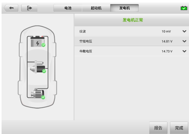
图 11-8 “发电机检测结果” 界面示图
