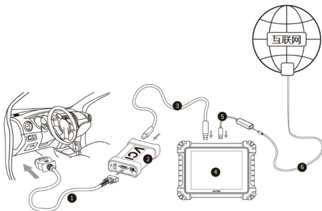
图 18-1 “远程专家”技师端连接示意图
