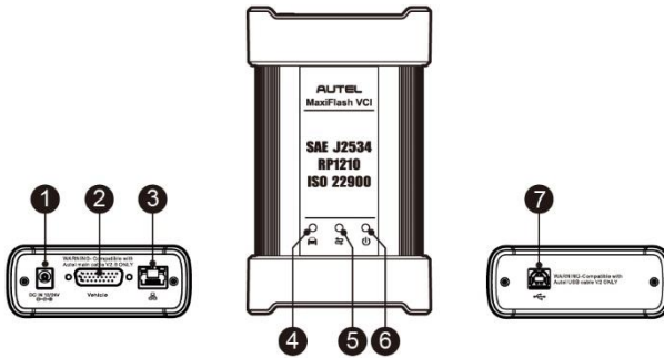
图 2-4 MaxiFlash VCI 编程设备
