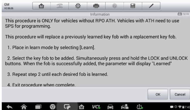
图 5-30 示例 IMMO 注释屏幕
