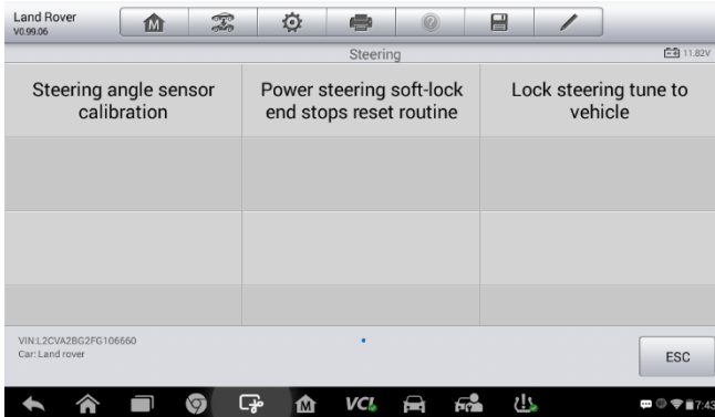
图 5-18 SAS 功能菜单示例
