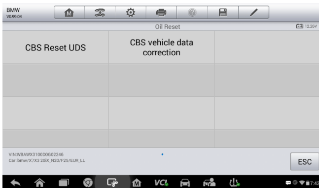
图 5-1 机油复位功能列表
