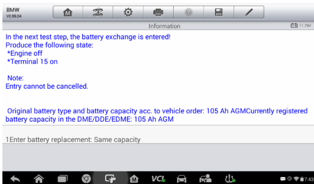
图 5-14 样品 BMS 屏幕 5
